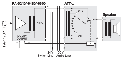
Noodbericht/voorrangsrelais
