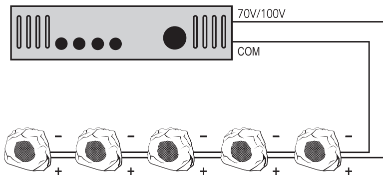
5 diffusori collegati in parallelo con terminale del trasformatore a 16W
