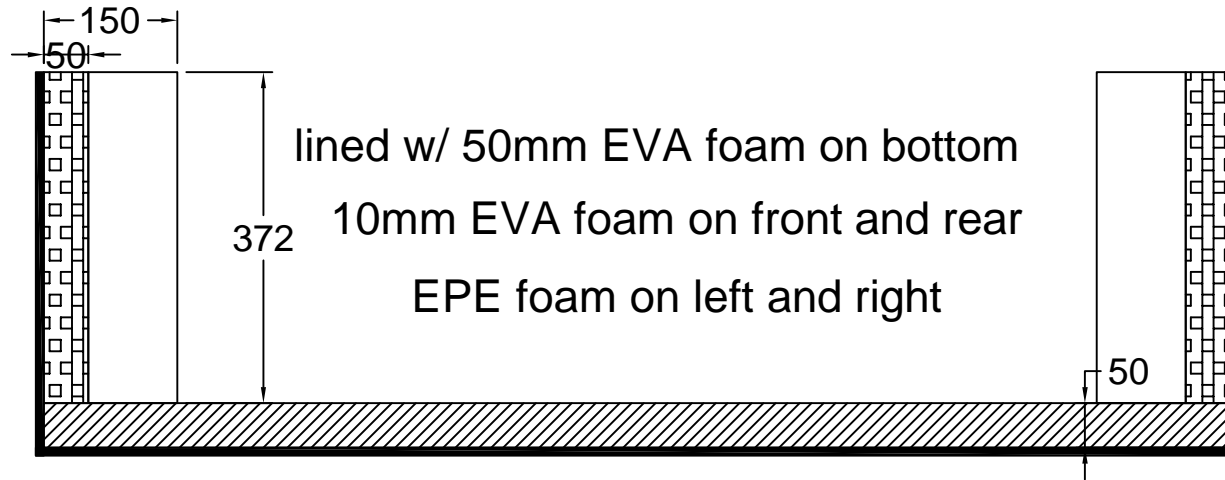
A-A VIEW
