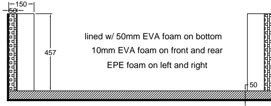
A-A VIEW
