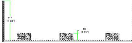
A-A VIEW
