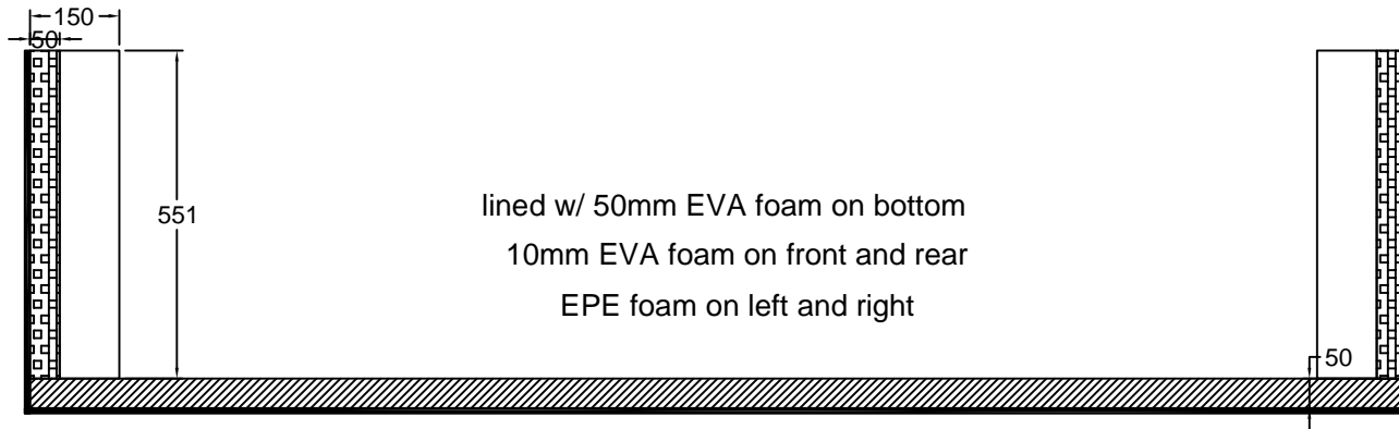
A-A VIEW
