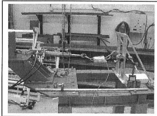
Traction sur le milieu de l'équerre
