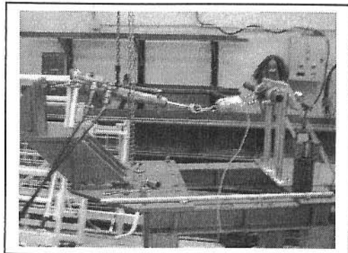
Traction sur le haut de l'équerre
